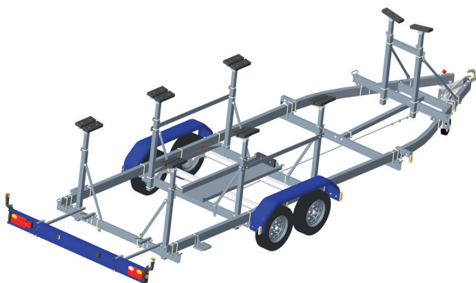
GS13V avec kit voilier
